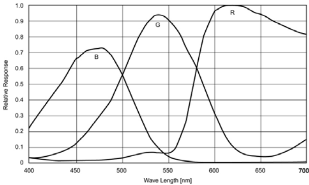
DX 40 – 285 GigE
